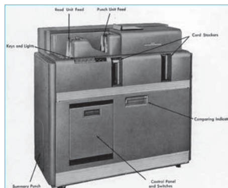
reproductrice IBM 519 (1949)
